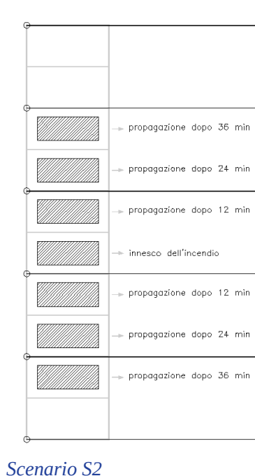
Illustrazione V.6-2: Schematizzazione degli scenari di incendio di progetto
