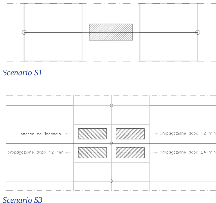
Illustrazione V.6-2: Schematizzazione degli scenari di incendio di progetto
