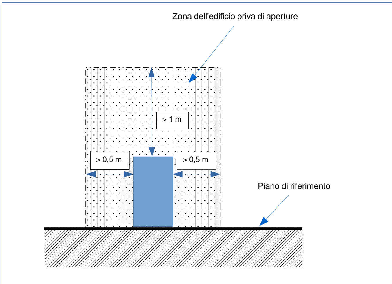
Tavola 4 - installazione all'aperto adiacente a parete
